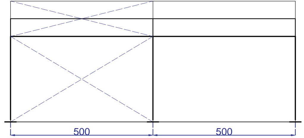
YAN GÖRÜNÜŞ
