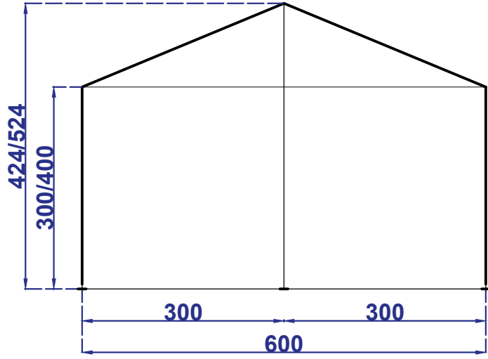
ÖN GÖRÜNÜŞ
