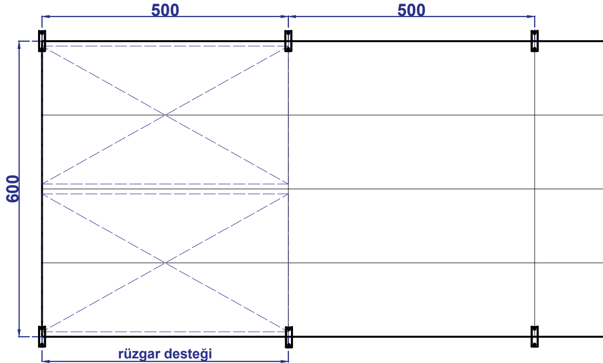
TEPE GÖRÜNÜŞÜ
